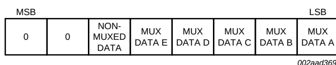
Fig 5. I 2 C-bus MUX_OUTx data byte
