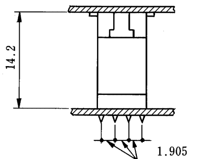
FX2C(A)2-*P-1.27DSA(L)
