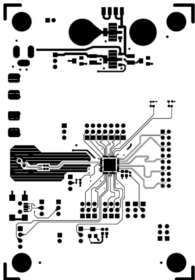
Top Layer
