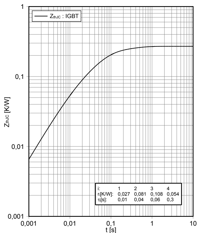
Transienter Wärmewiderstand IGBT, Brems-Chopper transient thermal impedance IGBT, Brake-Chopper
