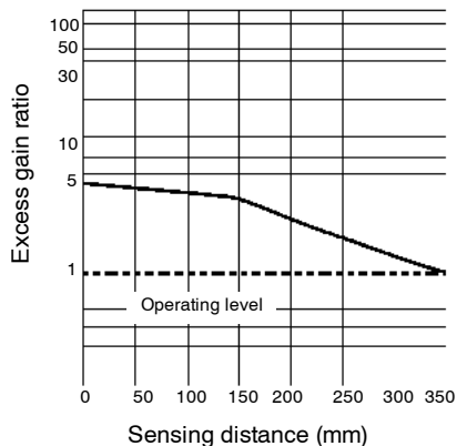
E32-UDAT1-3F with E3X-A11 amplifier
