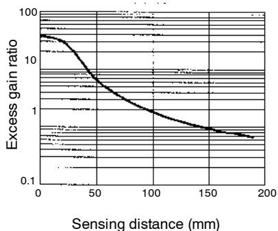
E32-UDBT1-3F with E3JU-X amplifier
