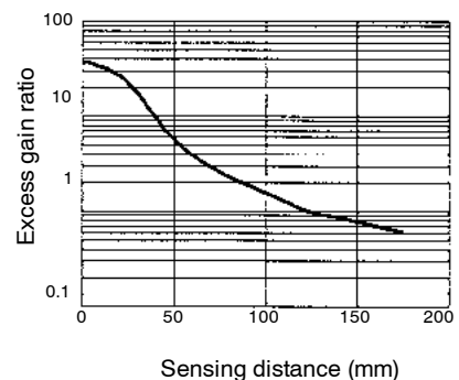
E32-UDBT1-6F with E3JU-X amplifier
