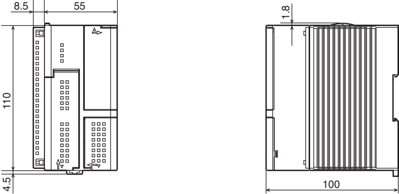
CPU Module
