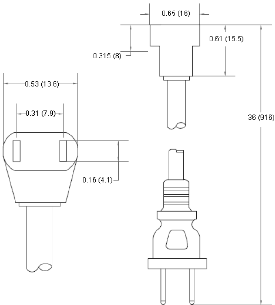
Dimensions : Inches (Millimetres)
