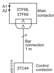
3TF6. 33-Q..
