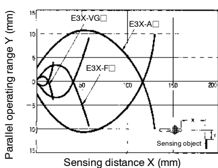
E32-D11L with E3X-A, E3X-F, and E3X-VG amplifiers
