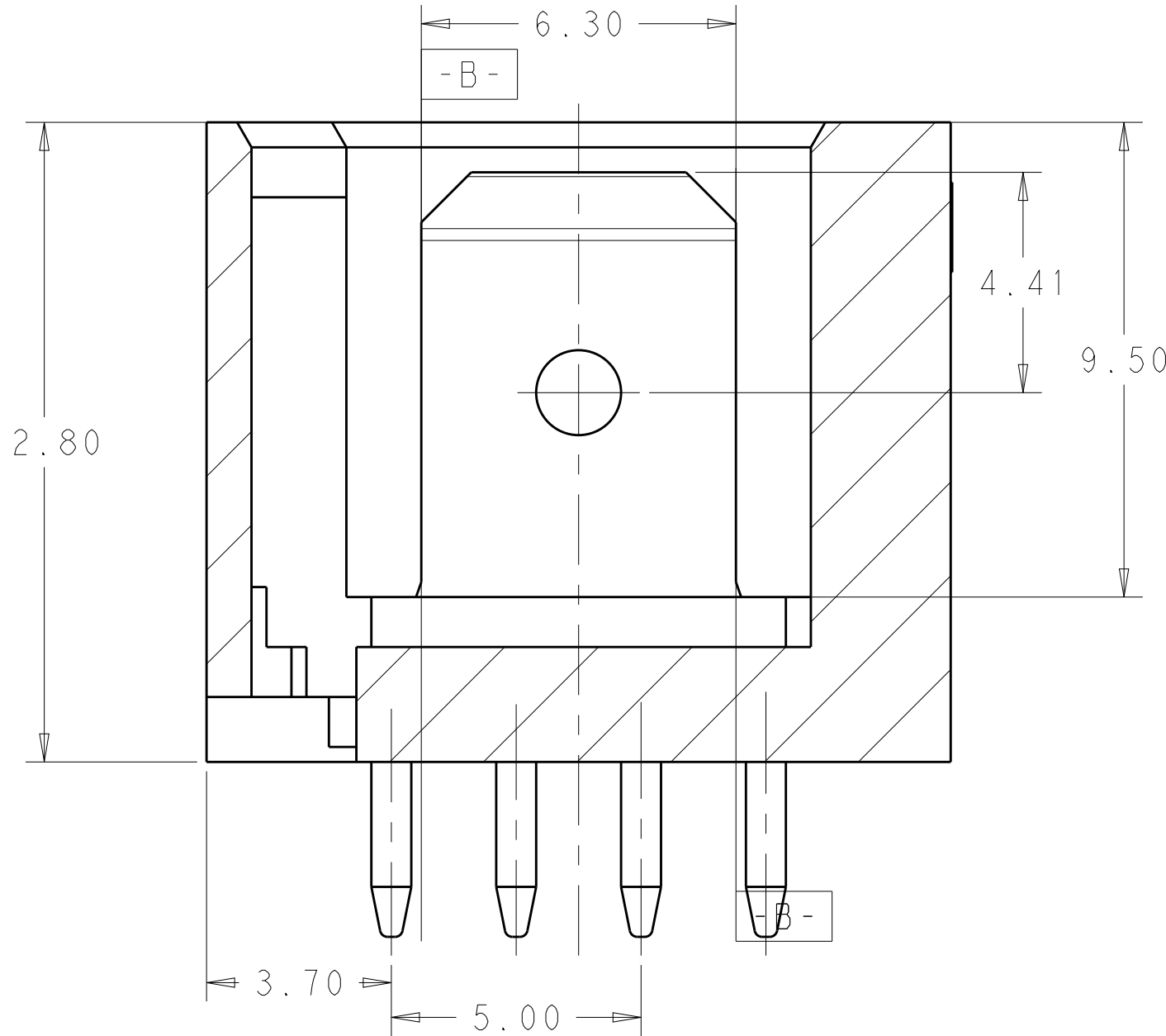
SECTION A-A
