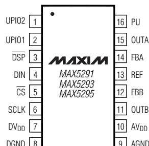
16 TSSOP
