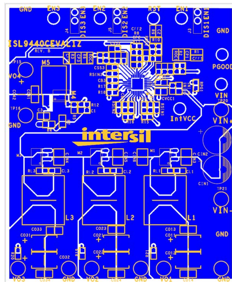
FIGURE 16. TOP LAYER
