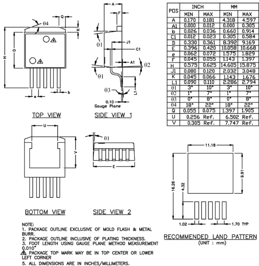
TO-263-5 (U)
