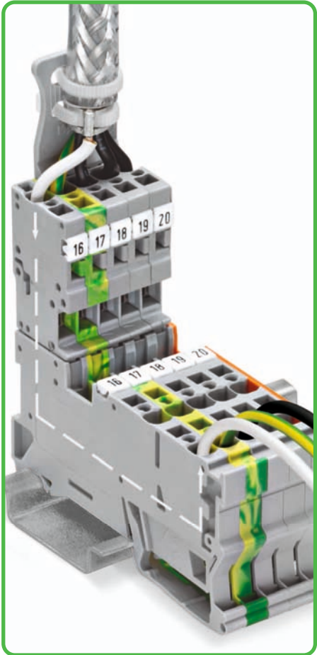
Schirmübergabe hier am Beispiel einer X-COM®-Steckverbindung
