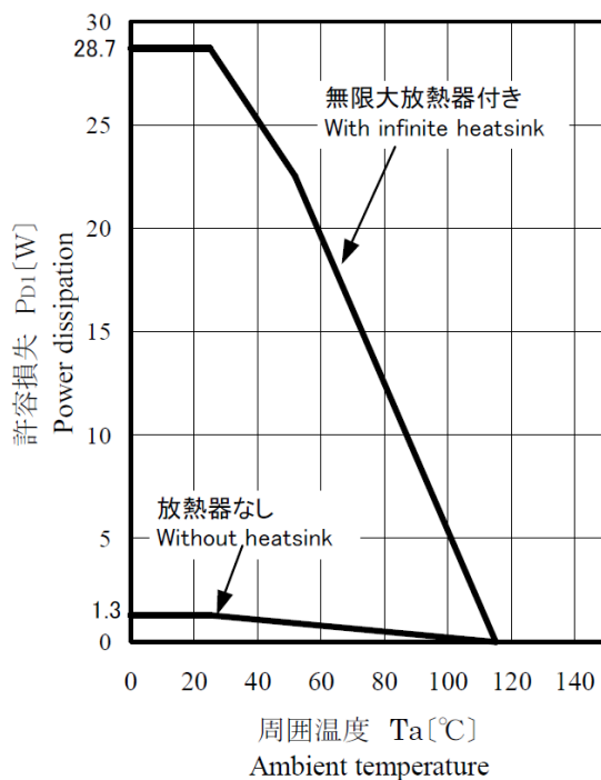
STR-W6735N MOSFET T_a - P_{D1} 曲線 curve
