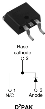
D²PAK
