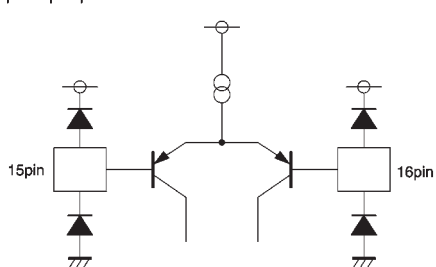
Op-amp input
