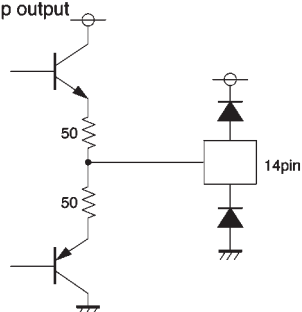
Op-amp output
