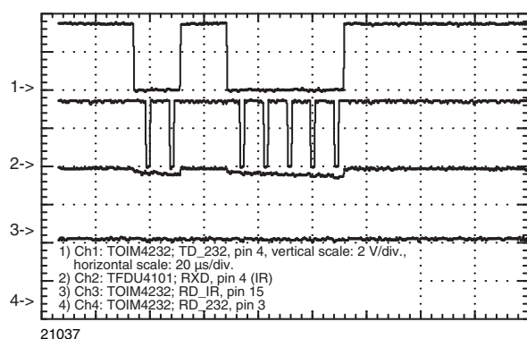
Fig. 11 - Echo-Suppression
