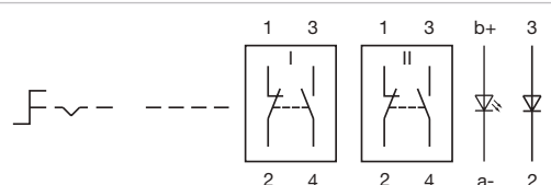
Wiring diagram 279
