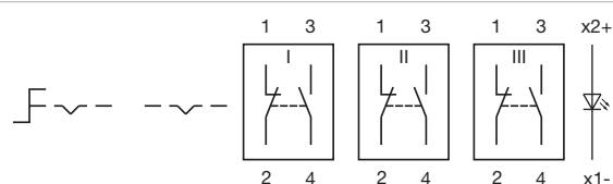
Wiring diagram 277
