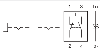
Wiring diagram 277
