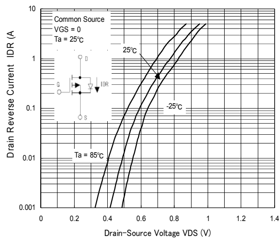
IDR - VDS
