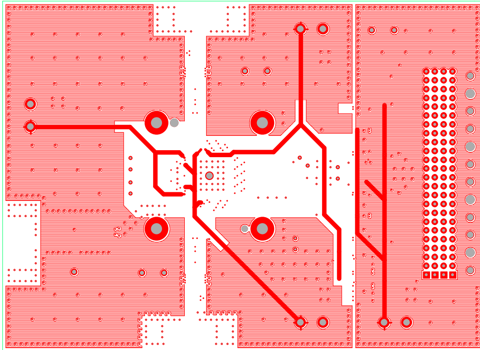
Layer 3: Power
