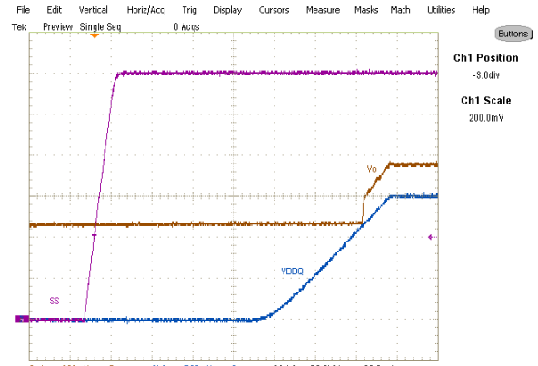
Fig. 8: Start up with Prebias, 0A Load Ch 1 :V out , Ch 2 :V DDQ , Ch 3 :SS
