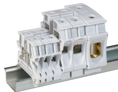
0371 60 + 0371 61 + 0371 62 + 0371 63 + 0371 64 + 0371 65 + 0371 66
