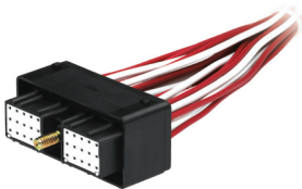
Connector 18 pos.
