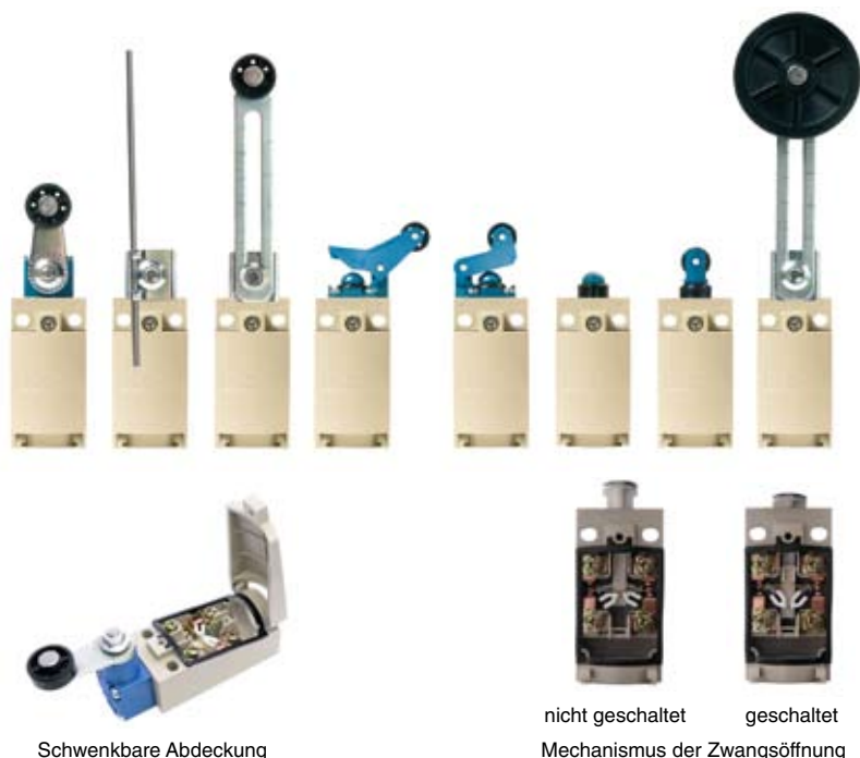
Schwenkbare Abdeckung
