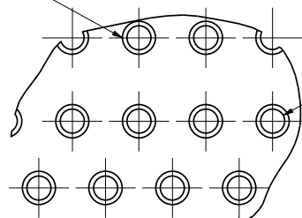
DETAIL E SCALE 5.000
