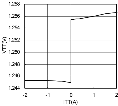
Fig.8 ITT-VTT (DDR- I )
