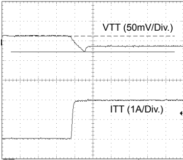
Fig.3 DDR II (-1A→1A)
