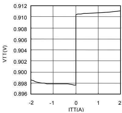
Fig.9 ITT-VTT (DDR- II )
