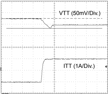
Fig.1 DDRI (-1A→1A)
