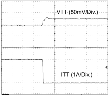
Fig.2 DDRI (1A→-1A)
