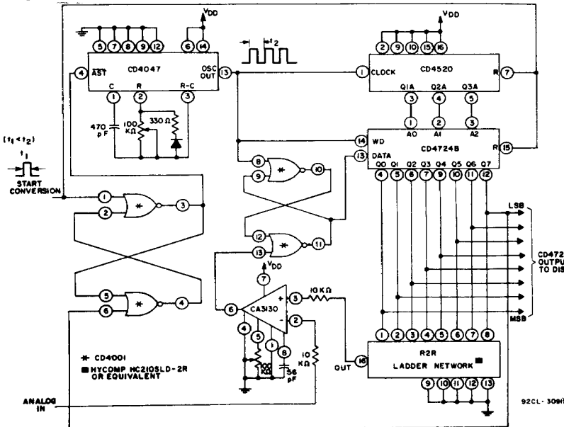
Fig. 5— A/D converter
