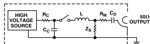
Figure 12. EFT Generator
