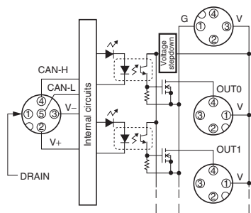
DRT2-OD04CL (NPN)
