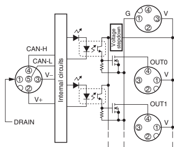
DRT2-OD08CL (NPN)
