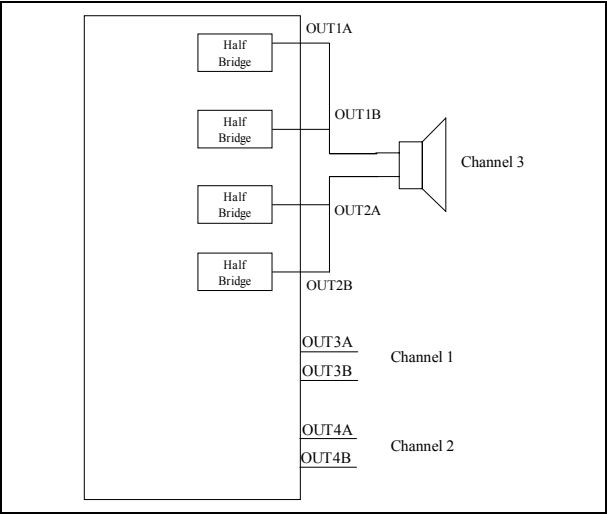
OCFG = 11
