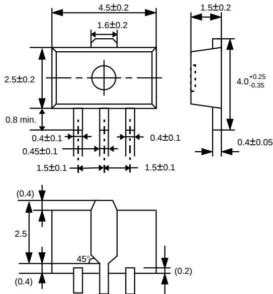
(3) SOT-89-3
