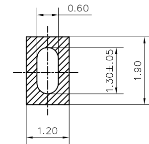
DETAIL A 5 : 1
