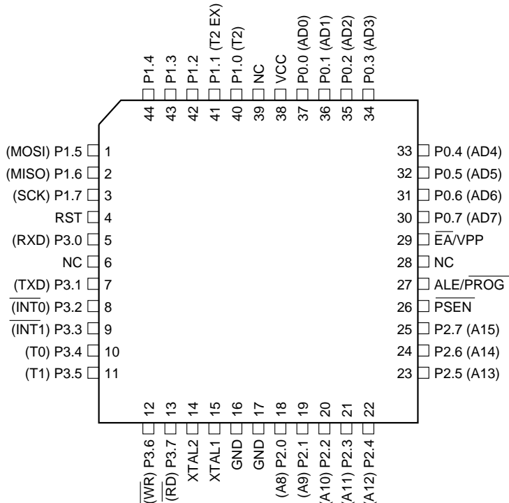
TQFP
