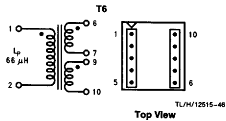
FIGURE 28. Schott 67140900
