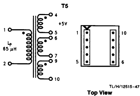
FIGURE 29. Schott 67140890
