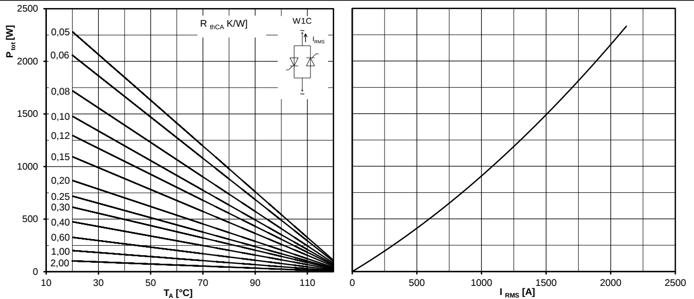
Höchstzulässiger Effektivstrom / Maximum rated RMS current I_{RMS}
