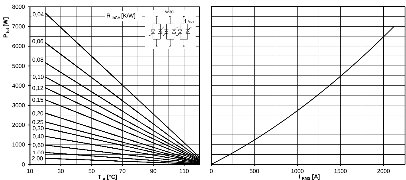
Höchstzulässiger Effektivstrom / Maximum rated RMS current I_{RMS}
