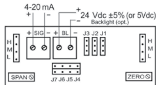
WIRING
