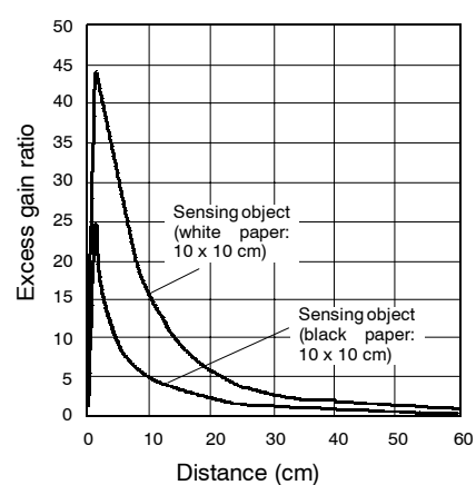
E3F2-DS30□4 E3F2-DS30□4-P1
