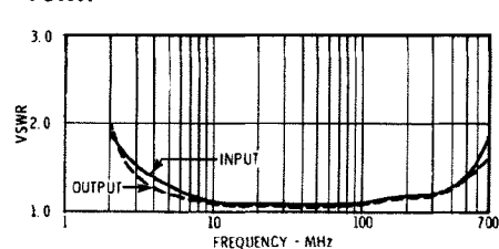
VSWR
