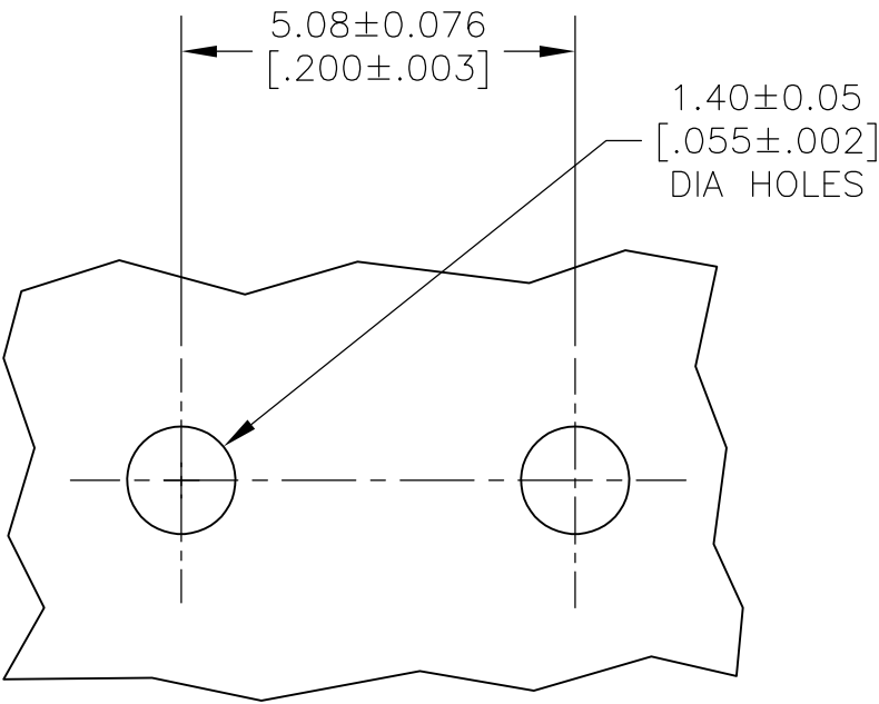
P.C.BOARD HOLES
