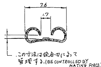
断面 A-A 実寸 8-1 (SECT) (SCALE)
