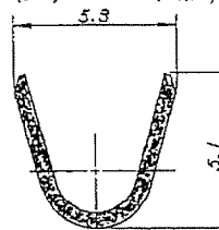
断面 B-B 実寸 8-1 (SECT) (SCALE)
