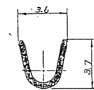
断面 B-B 実寸 8-1 (SECT) (SCALE)
