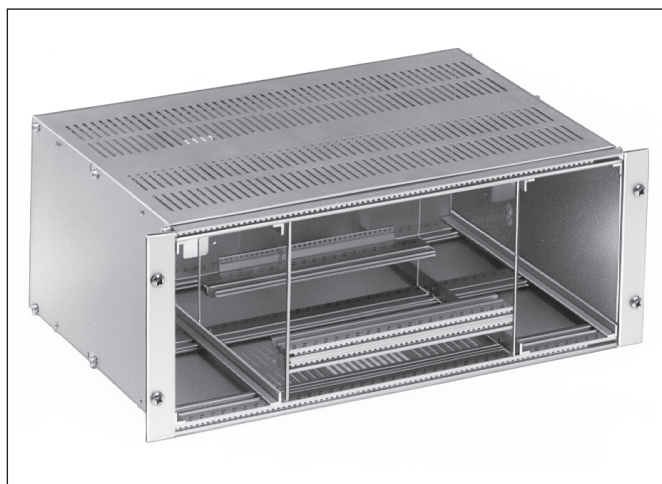
4 HE Sonderbaugruppenträger Special Subrack 4 U Rack modulaire spécial 4 UH
