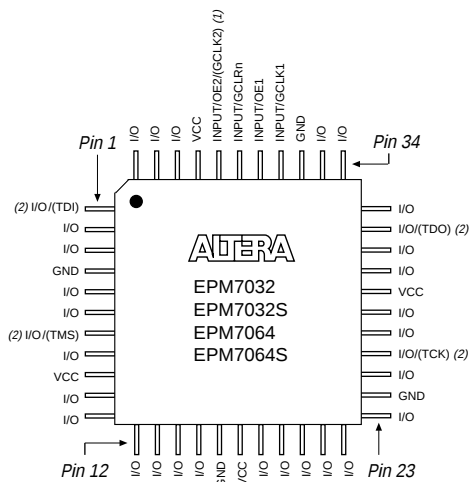
44-Pin TQFP
