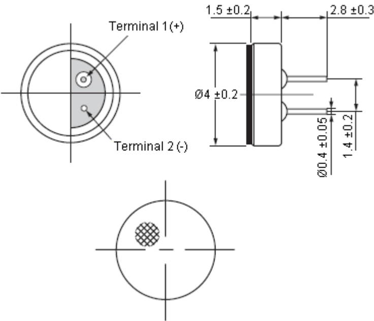
Dimensions : Millimetres
