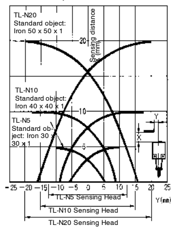
TL-N□ME, TL-N□MY
