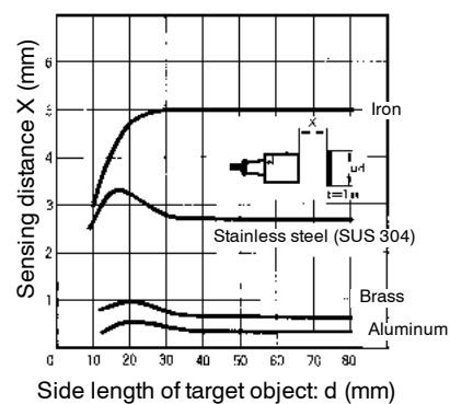
TL-N5
