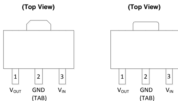
SOT-89 (Option 1)
