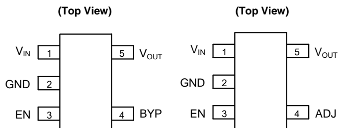
SOT-23-5
