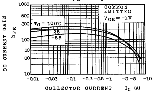
h_{FE} - I_C
