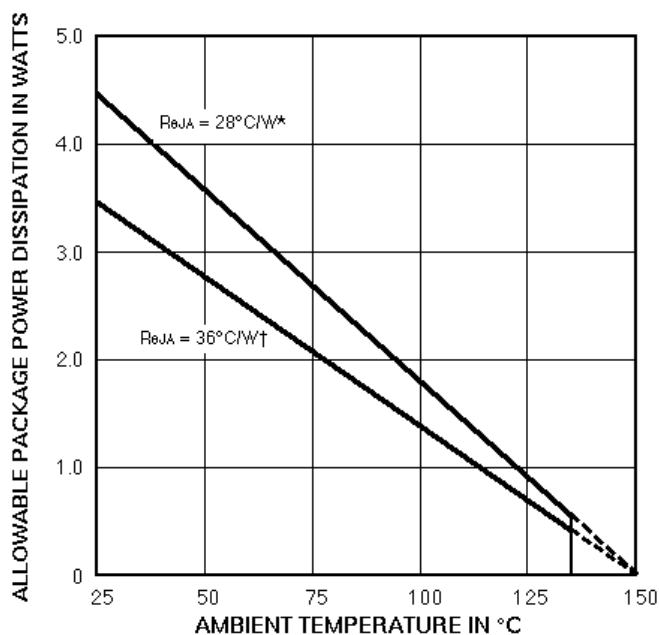
A3940KLP (TSSOP)
