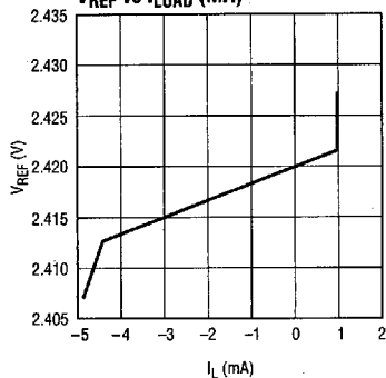
VREF vs ILOAD (mA)
