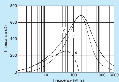
BLM18AG601SZ1/BLM18AG601SH1
