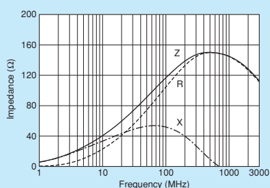
BLM18EG121SZ1/BLM18EG121SH1
