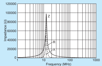
NFZ32BW881HZ10
