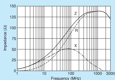
BLM18EG101TZ1/BLM18EG101TH1
