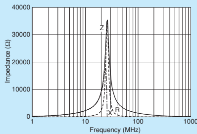
NFZ32BW221HZ10
