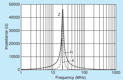
NFZ32BW291HZ10
